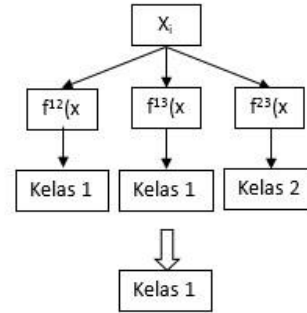
Gambar 2.6 Contoh klasifikasi dengan menggunakan metode OAO
