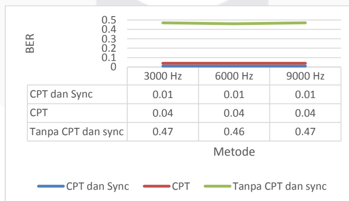
Gambar 4.1 Pengaruh CPT dan sync terhadap serangan LPF
