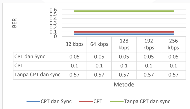
Gambar 4.7 Pengaruh CPT dan sync terhadap serangan Mp4 Compression
