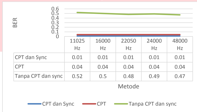
Gambar 4.2 Pengaruh CPT dan sync terhadap serangan Resampling
