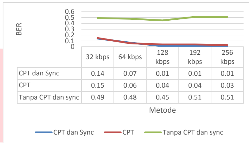
Gambar 4.4 Pengaruh CPT dan sync terhadap serangan Mp3 Compression
