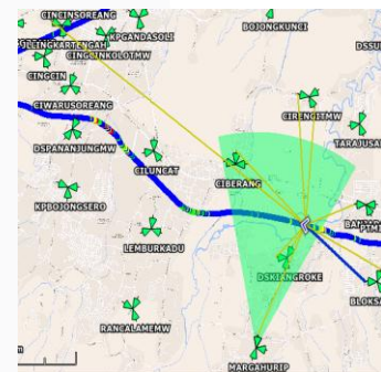
Gambar 3.8 Serving Site di Area Bad Ec/No
