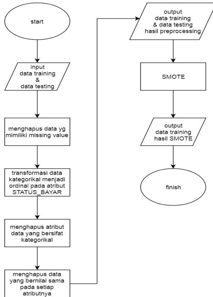
Gambar 2 Tahap Preprocessing
