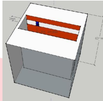
Gambar 1 Sensor Kapasitif
