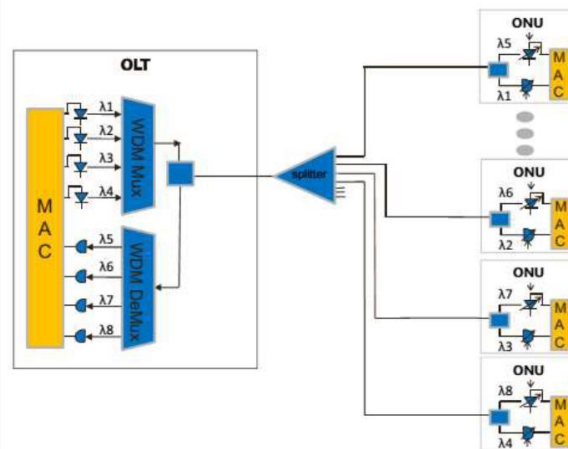
Gambar 1 Arsitektur TWDM-PON [3]
