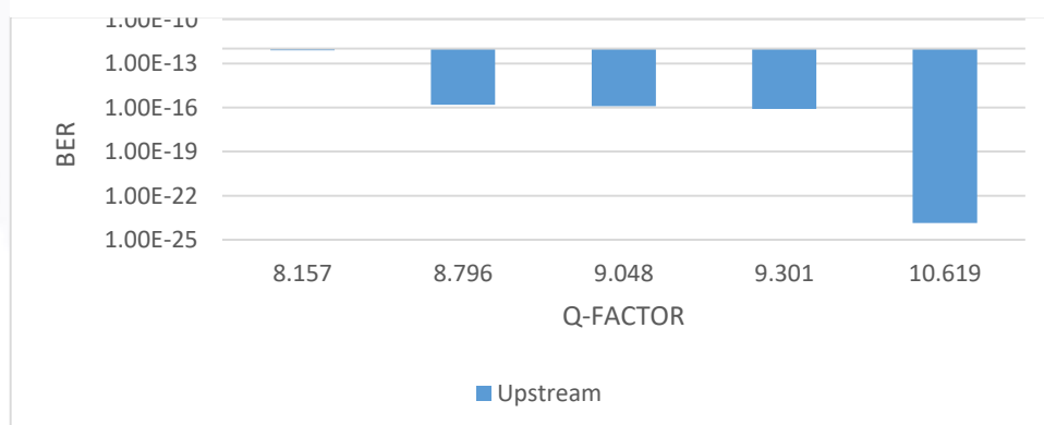
Gambar 6 Hasil Q-factor dan BER Upstream Skenario 1
