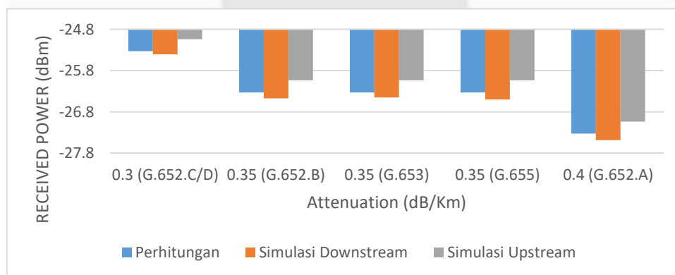
Gambar 3 Hasil LPB Skenario 1
