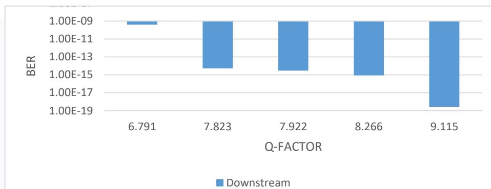
Gambar 5 Hasil Q-factor dan BER Downstream Skenario 1
