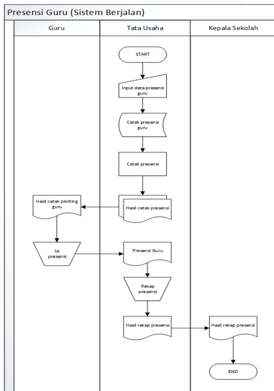
Gambar 3. 4 Flowmap Presensi Guru yang berjalan
