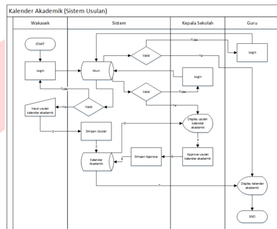
Gambar 3. 3 Flowmap Kalender Akademik yang diusulkan
