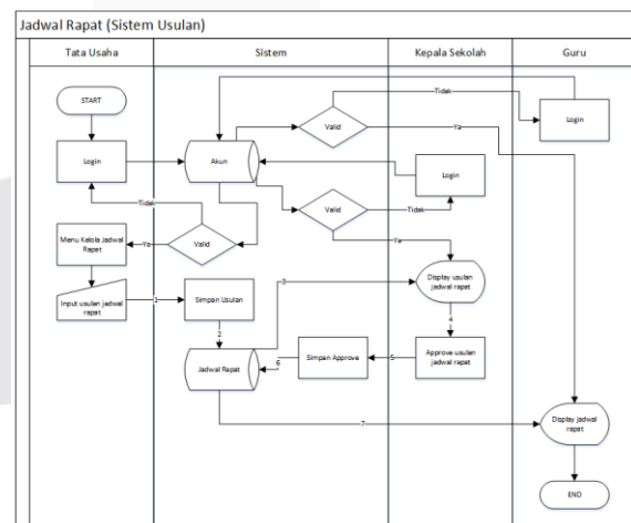
Gambar 3. 4 Flowmap Undangan Rapat yang diusulkan
