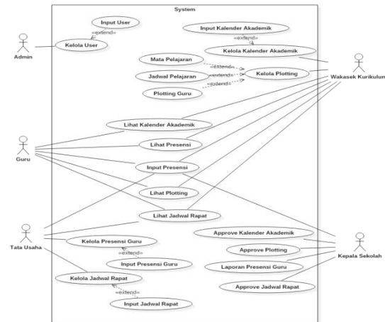
Gambar 3. 9 Use Case Diagram yang diusulkan
