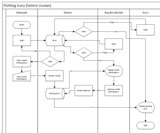
Gambar 3. 6 Flowmap Plotting Guru yang diusulkan
