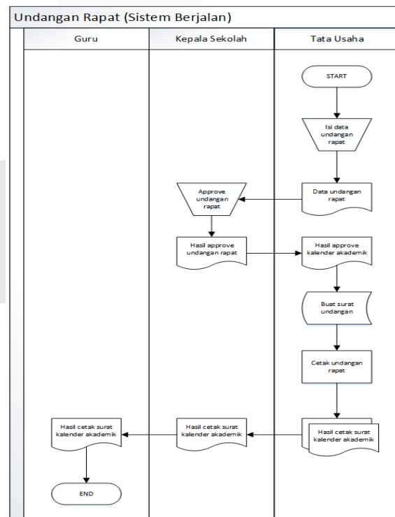
Gambar 3. 1 Flowmap Undangan Rapat yang berjalan
