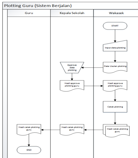
Gambar 3. 2 Flowmap Plotting Guru yang berjalan
