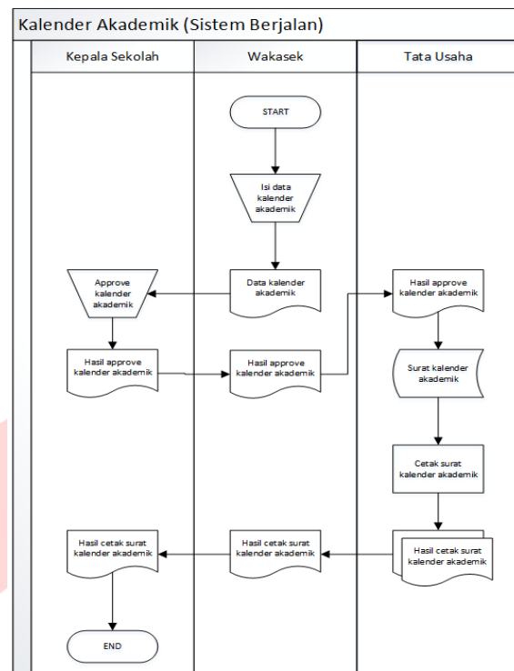
Gambar 3. 1 Flowmap Kalender Akademik yang berjalan
