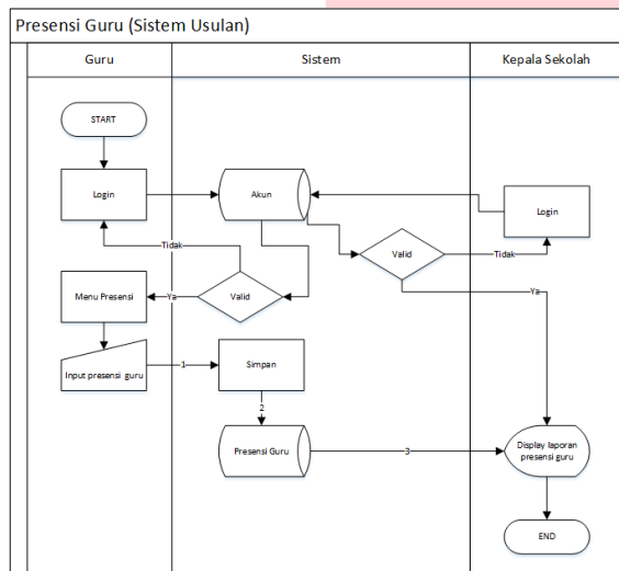
Gambar 3. 5 Flowmap Presensi Guru yang diusulkan
