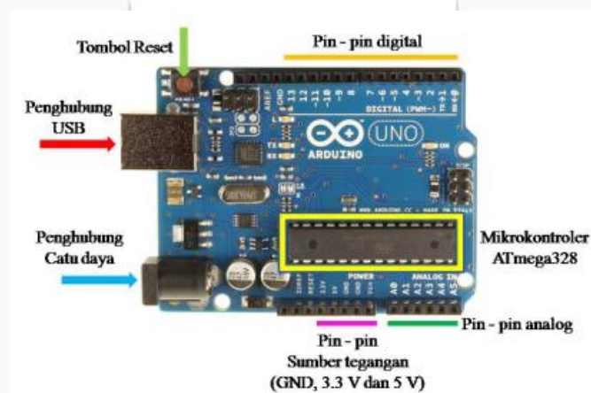
Gambar 2. Arduino Uno[6]
