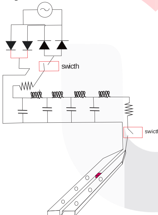
Gambar 2.6 Prototipe plan
