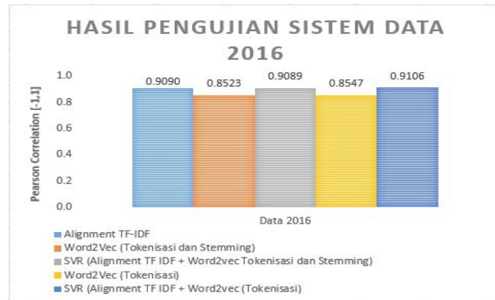
Gambar 9: Hasil Pengujian Sistem Menggunakan data Alquran 2016
