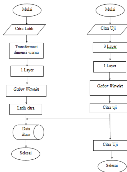
Gambar 3.2 Diagram Alir Proses Identifikasi Tekstur pada Keju
