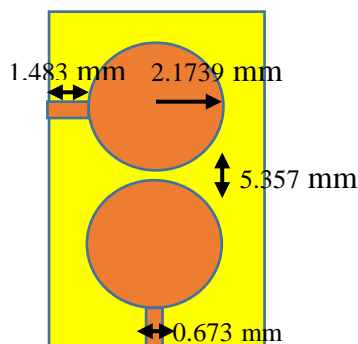
Gambar 2. Tampak Depan
