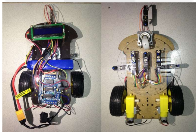
Gambar 3.4 Implementasi Robot
