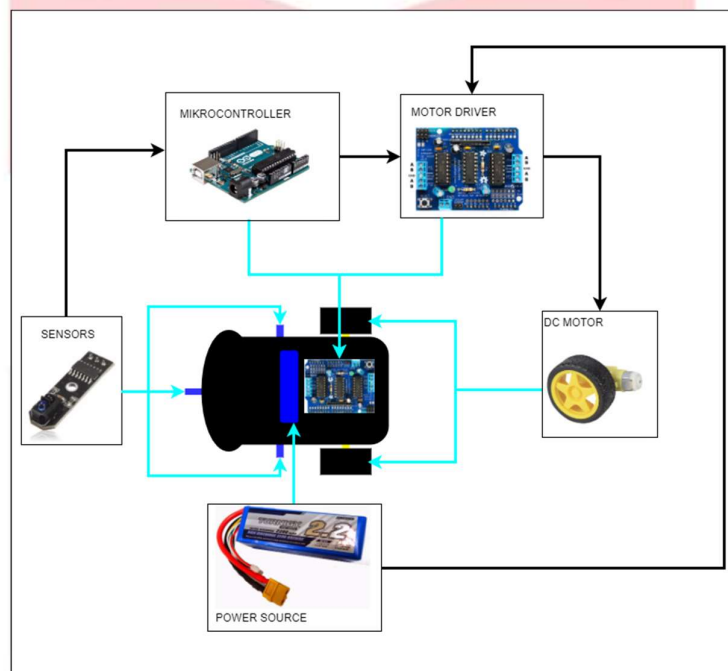
Gambar 3.1 Diagram Umum Sistem
