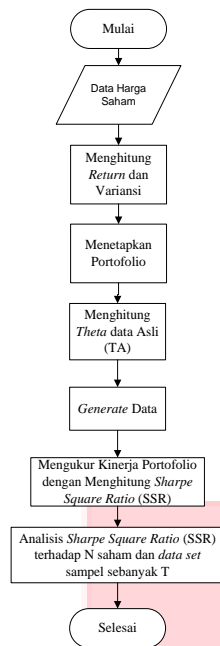
Gambar 3.1 Flowchart Sistem kinerja portofolio menggunakan Sharpe Square Ratio (SSR)
