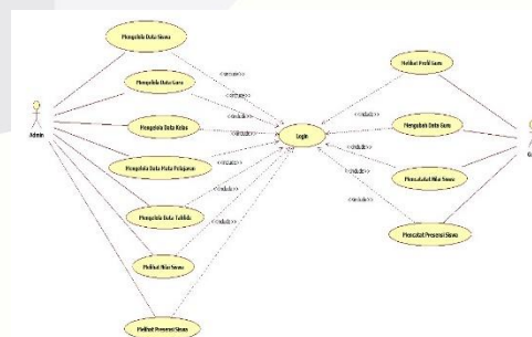
Gambar 3.2 Diagram Use Case Aplikasi Pencatatan Nilai dan Presensi untuk Web
