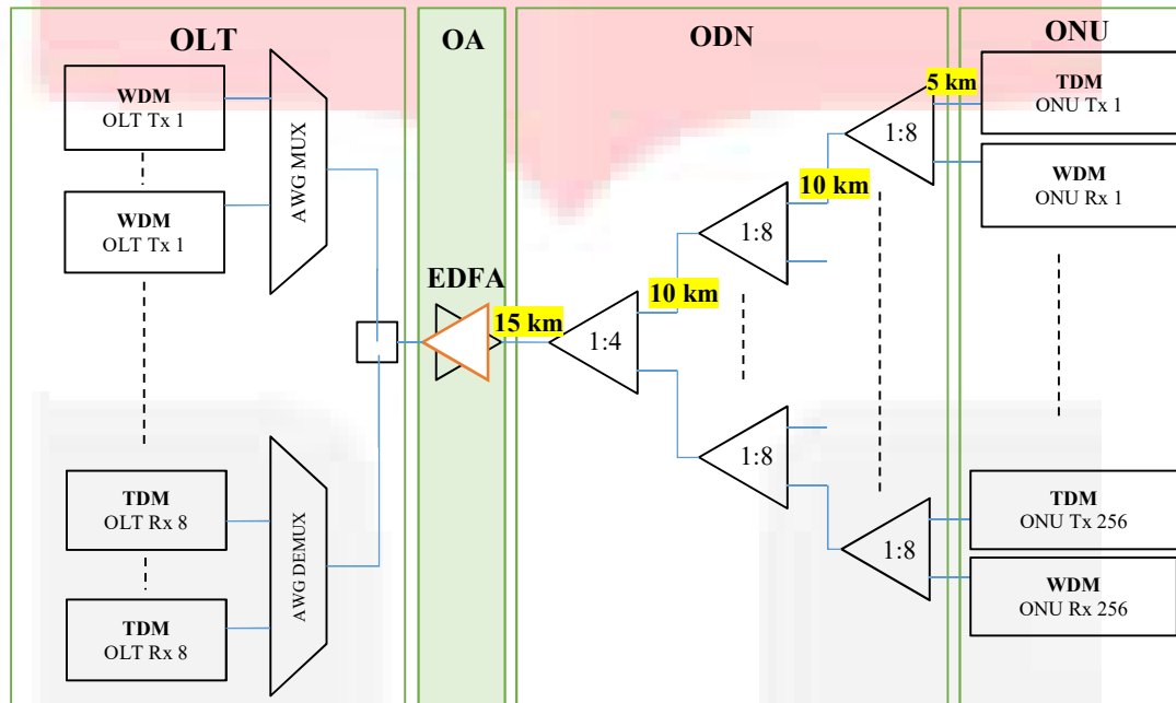
Gambar 3 Sistem TWDM-PON
