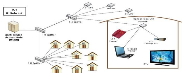
Gambar 2.1 Arsitektur FTTH
