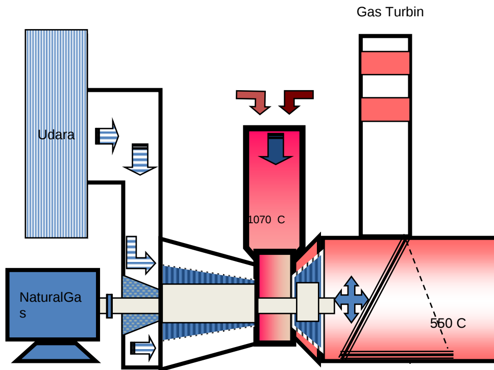
Gambar 1.4 Diagram Pembangkit Listrik Tenaga Gas
