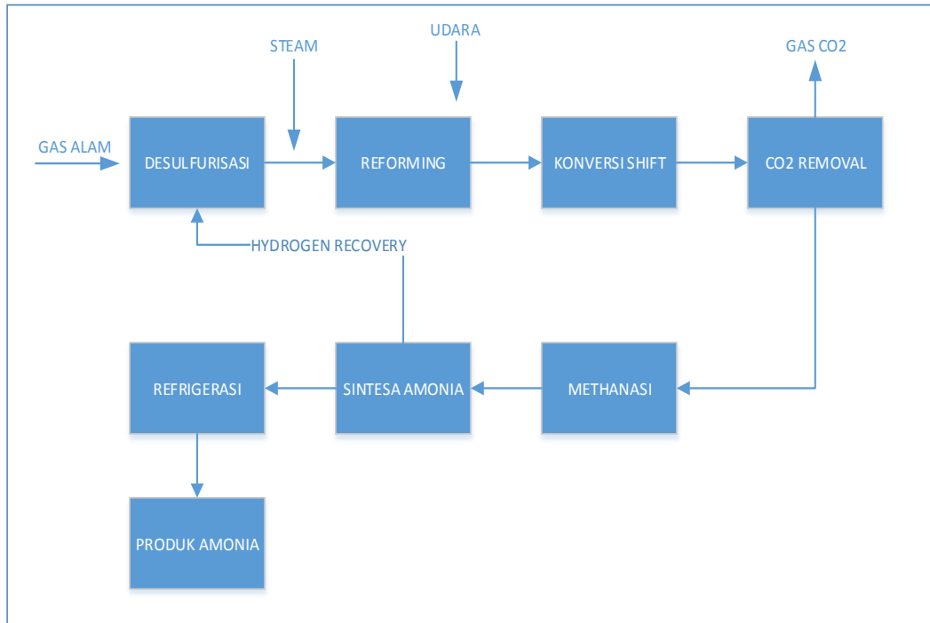
Gambar I.3 Diagram Blok Pembuatan Ammonia
