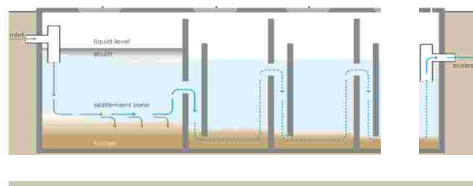
Gambar 2.2 Proses aliran pada Anaerobic Baffled Reactor 3 sekat
