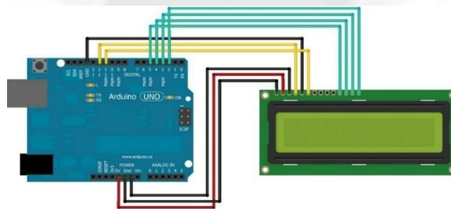
Gambar 3.8 Konfigurasi Arduino ke LCD
