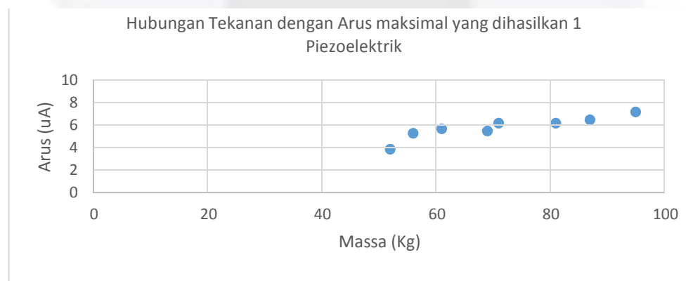
Gambar 4.4 Hubungan nilai arus yang dihasilkan oleh 1 piezoelectric dengan variasi beban penguin
