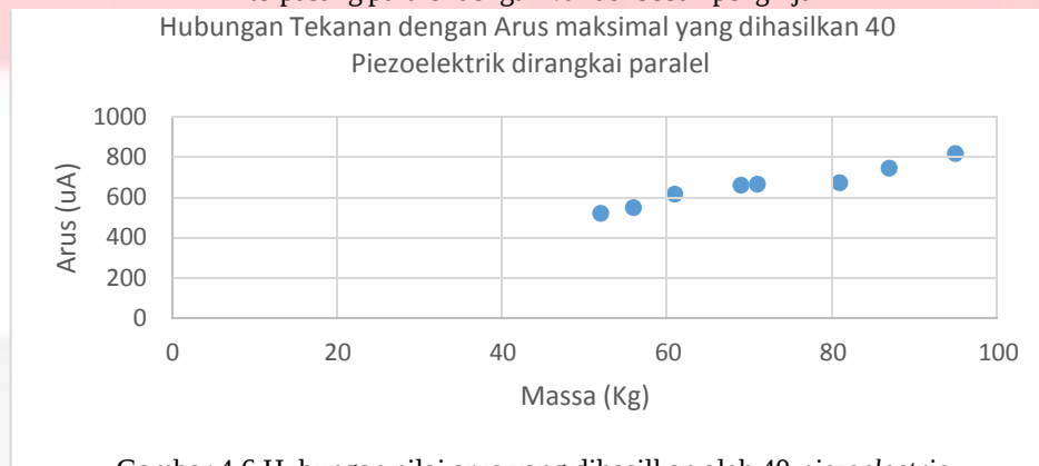
Gambar 4.6 Hubungan nilai arus yang dihasilkan oleh 40 piezoelectric terpasang paralel dengan variasi beban penguinjak
