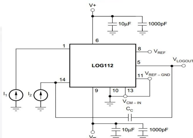
Gambar 3.7 Rangkaian Sensor Arus menggunakan IC Log112
