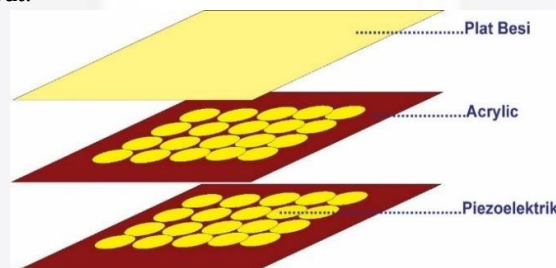
Gambar 3.2 Konstruksi Modul Piezoelectric
