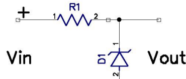
Gambar 3.5 Rangkaian dioda zener
