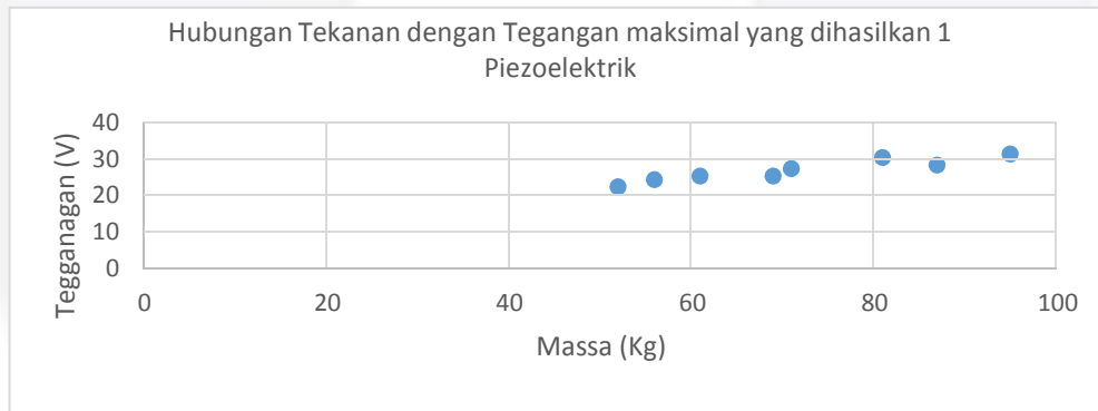
Gambar 4.3 Hubungan nilai tegangan yang dihasilkan oleh 1 piezoelectric dengan variasi beban penguin
