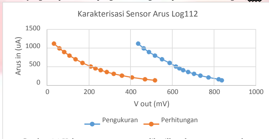
Gambar 4.1 Hubungan tegangan yang dihasilkan dengan arus masukan
