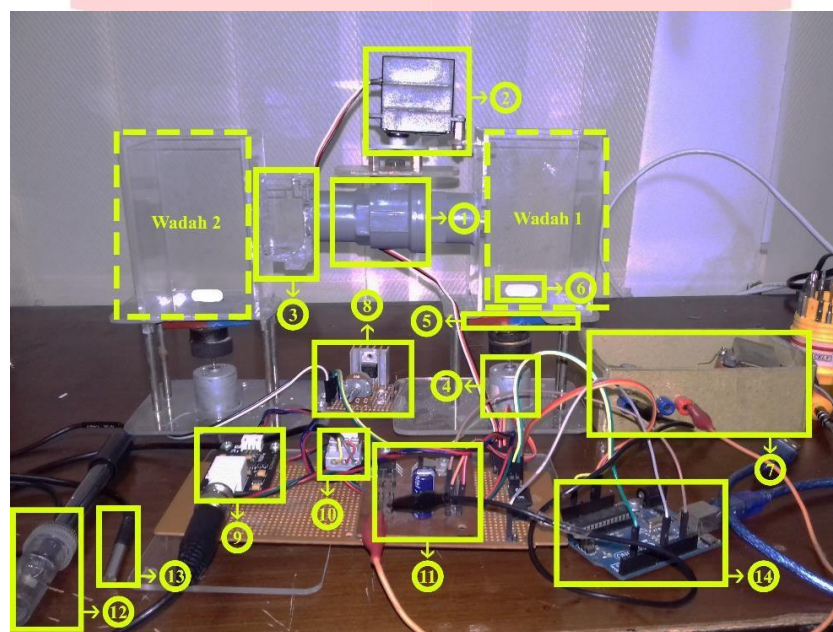
Gambar 4. Hasil perancangan alat
