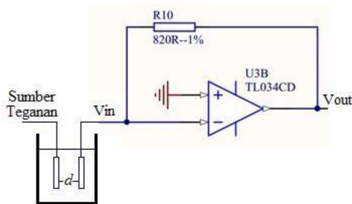
Gambar 2 Rangkaian Penguat Tegangan Conductivity meter
