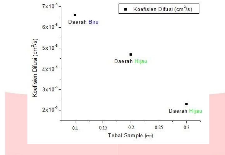
Gambar 4.10 Nilai koefisien difusi molekul NaCl terhadap masing-masing sample dengan ketebalan yang berbeda.
