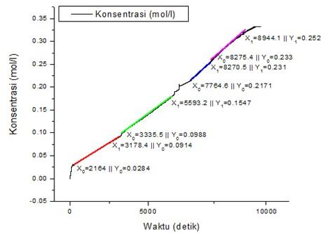
Gambar 7. Kurva perubahan konsentrasi terhadap waktu
