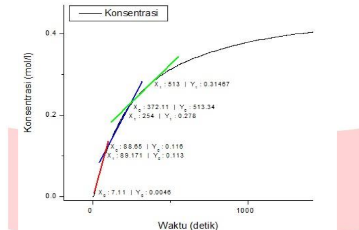
Gambar 6. Kurva perubahan konsentrasi terhadap waktu
