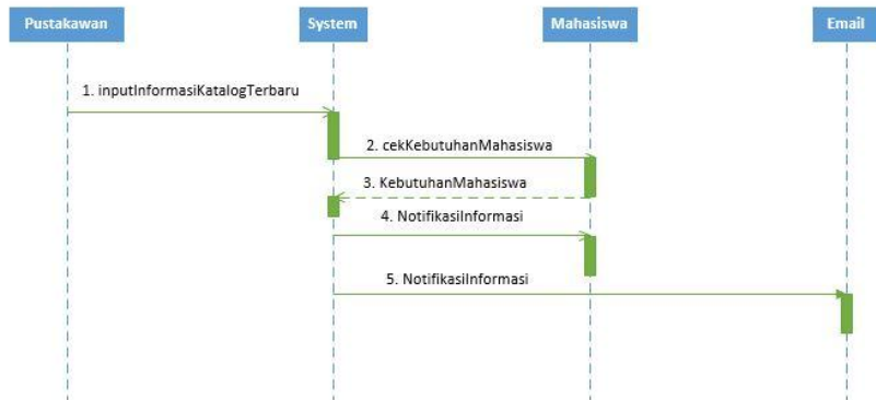
Gambar 4. 5 Pola Arsitektur Timeliness
