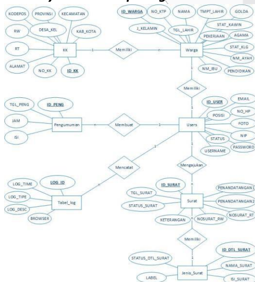
Gambar 6. ERD
