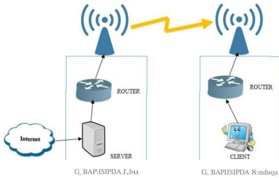
Gambar 2. Topologi Jaringan
