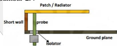
Gambar 2.4 Antena PIFA[4]
