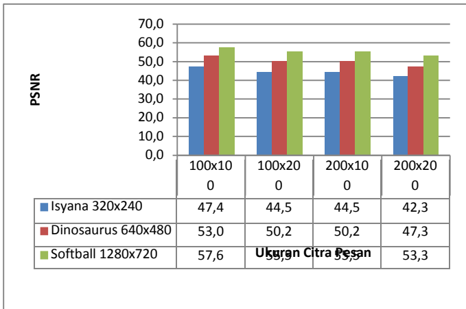
(a) Pengaruh ukuran cover dan ukuran citra pesan terhadap nilai PSNR (b) Pengaruh ukuran cover dan ukuran citra pesan terhadap nilai MSE
