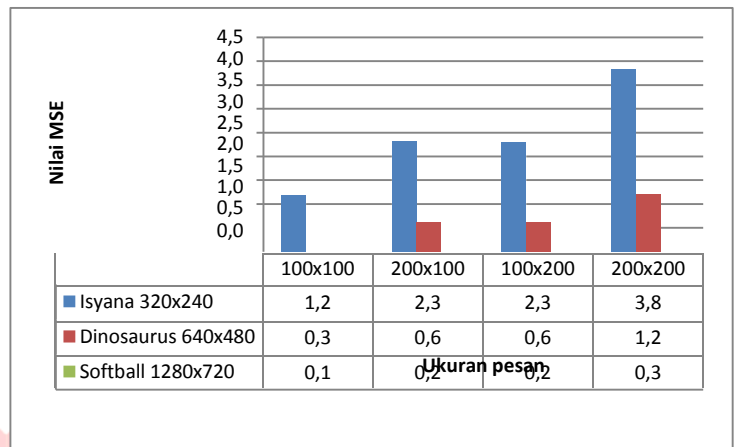
(a) Pengaruh ukuran cover dan ukuran citra pesan terhadap nilai PSNR (b) Pengaruh ukuran cover dan ukuran citra pesan terhadap nilai MSE
