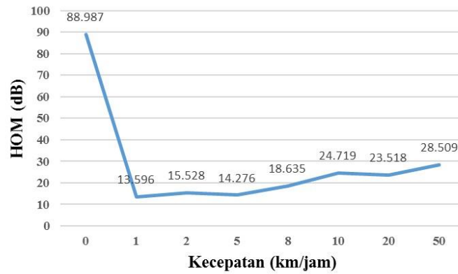
Gambar 3.2 Grafik Pengaruh Kecepatan terhadap HOM
