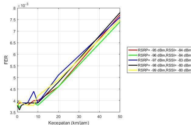
Gambar 3.3 Grafik Pengaruh Kecepatan terhadap FER
