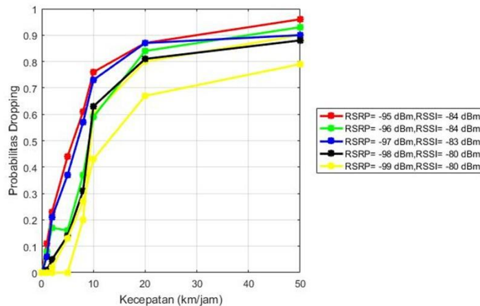
Gambar 3.1 Grafik Probabilitas Dropping
