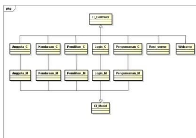
Gambar 3-4 Diagram kelas
