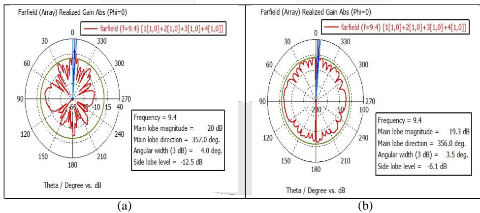
Gambar 4(f). Hasil Simulasi Pola Radiasi azimuth (a) Bada fasa 70° (b) Bada fasa 90° Berdasarkan hasil optimasi, antenna Array Mikrostrip 16 Elemen ditunjukkan pada tabel 4(a). yaitu :
