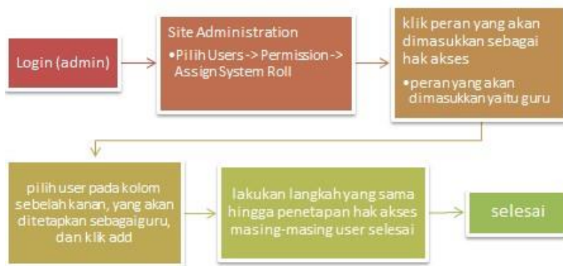
Gambar 7 Alur menetapkan peran (hak akses) masing-masing user
