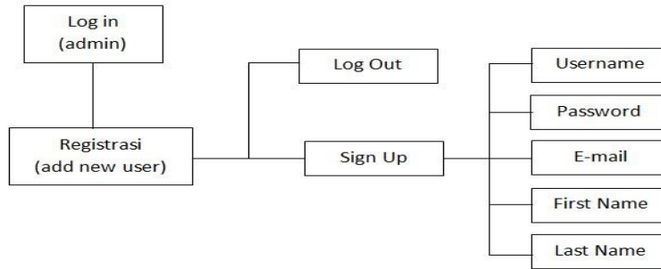
Gambar 3 Rancangan Skema Registrasi
