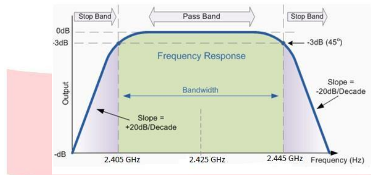
Gambar 2. Kurva BPF
