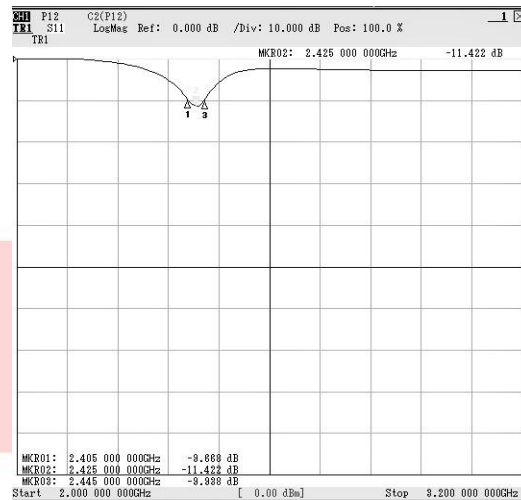
Gambar 7. Hasil pengukuran Return Loss (S11) pada filter
