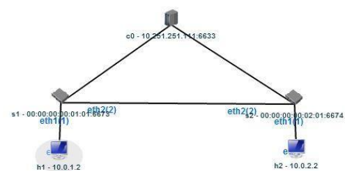
Gambar 2.5.7.a Topologi 2 switch
