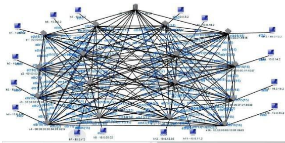
Gambar 2.5.7.d Topologi 16 switch
