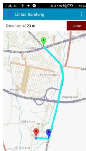
Gambar 5.4 Tampilan navigasi
