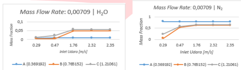
Gambar 7. Distribusi Fraksi H 2 O dan N 2 , MFR 0.00709 kg/s
