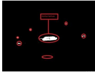
Gambar 3. Deteksi kontur
