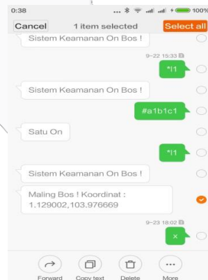
Gambar 4.4 Pilih titik koordinat dan copy
