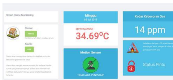
Gambar 11 Tampilan Halaman Web Terhadap Data Atribut Nomor 381
