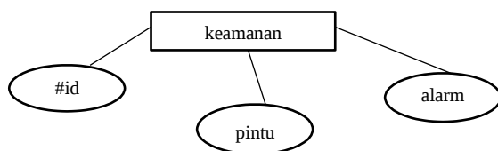
Gambar 2 ER-Diagram Keamanan
