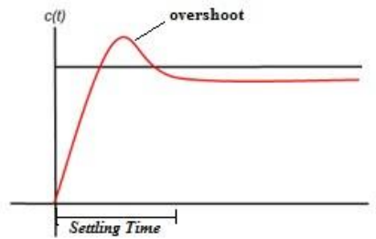
Gambar 3. Respon sistem
