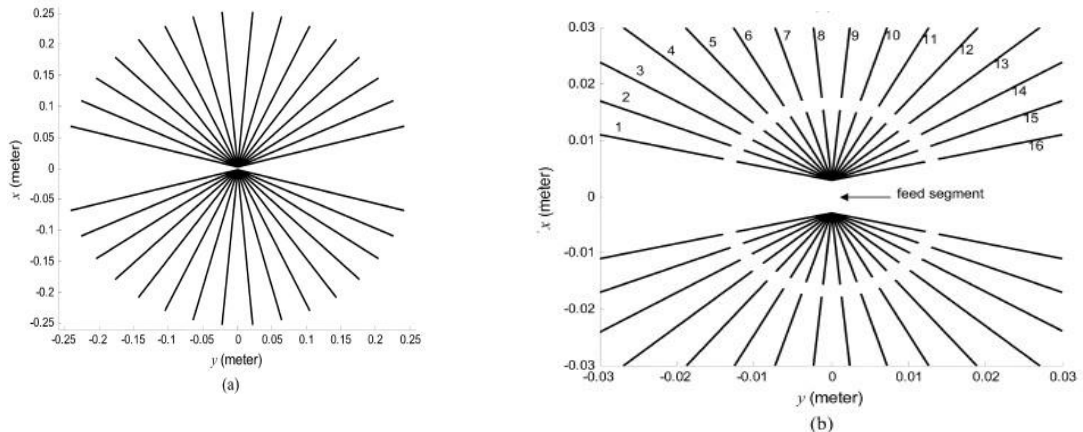
Gambar.2 (a) Geometri antenna wire bowtie , (b) geometri antenna dengan feed segment
