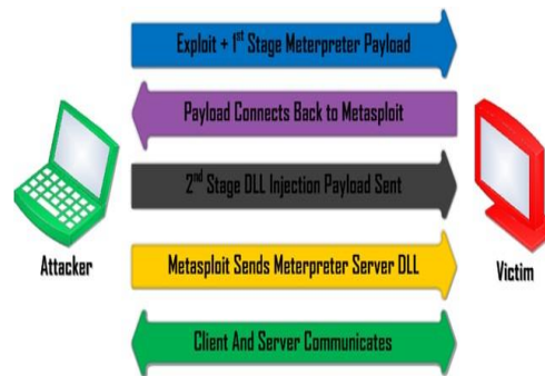
Gambar 2-4 Metasploit skema
