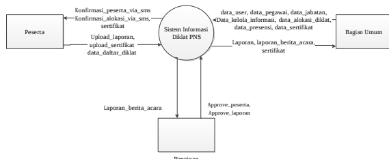
Gambar 2 Diagram Konteks
