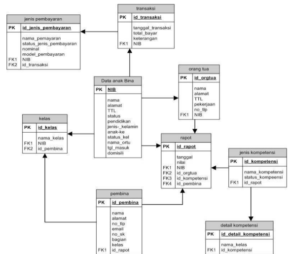
Gambar 5 Skema Relasi
