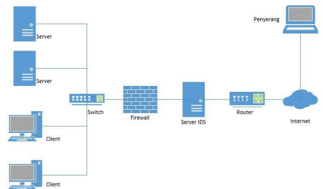
Gambar 2 Topologi jaringan dengan menggunakan IDS
