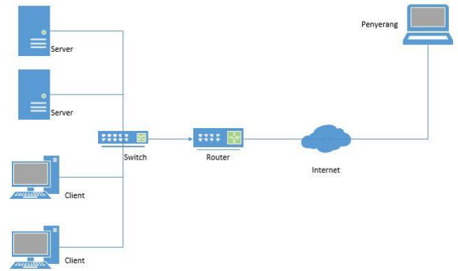
Gambar 1 Topologi jaringan tidak menggunakan IDS
