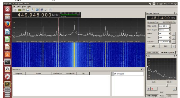
Gambar 4.3-3 Decode pada Modulasi AM
