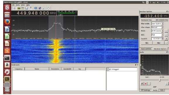
Gambar 4.5-2 Decode pada Modulasi WFM
