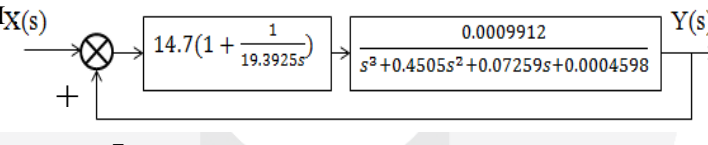
Gambar 3.3 Blok Diagram Sistem dengan Menggunakan Kontroler PI
