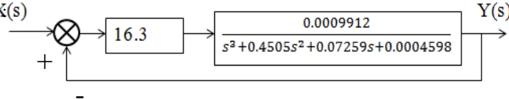
Gambar 3.2 Blok Diagram Sistem dengan Menggunakan Kontroler P
