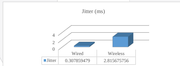
Gambar 4.6 Grafik Jitter pada Media Wired dan Wireless
