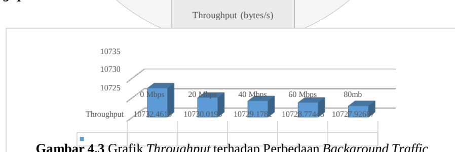
Gambar 4.3 Grafik Throughput terhadap Perbedaan Background Traffic
