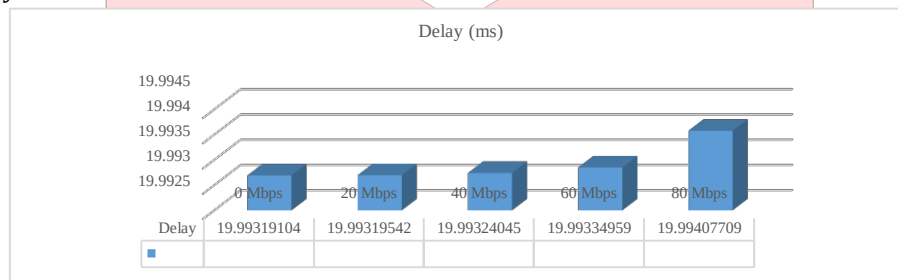
Gambar 4.1 Grafik Delay terhadap Perbedaan Background Traffic
