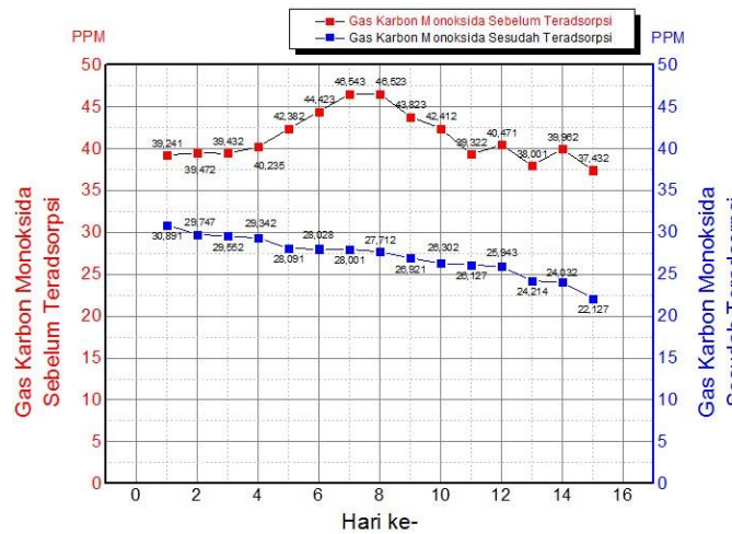
Gambar 8 Grafik Perubahan Gas Karbon Monoksida Sebelum dan Sesudah Terabsorpsi Filter Zeolite
