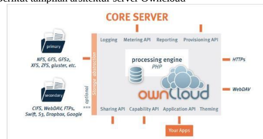
Gambar 4 Arsitektur Server Owncloud [6]
