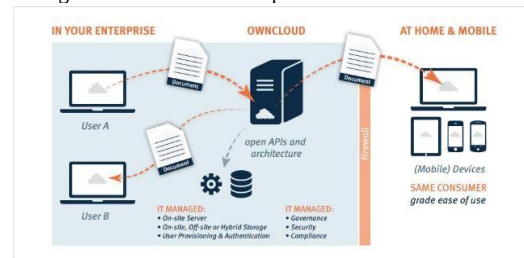
Gambar 2 Arsitektur Aktivitas Owncloud [6]
