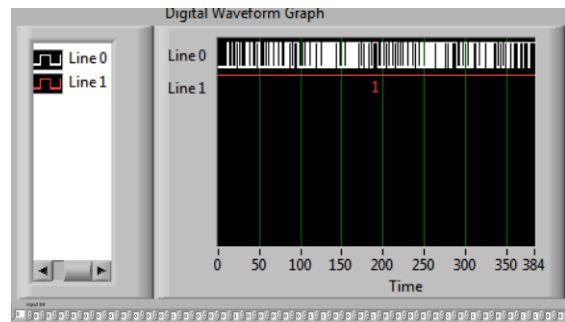
Gambar 4.4 Masukan Bit Termulasi 64 QAM
