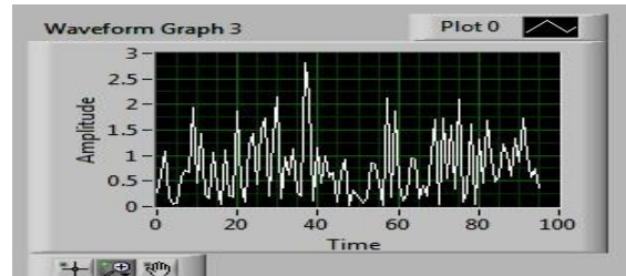
Gambar 4.3 Sinyal Termulasi 16 QAM + Noise
